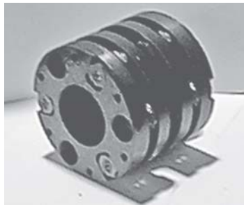
Муфта вспомогательного насоса смазки А9807-Л36
